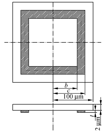
Fig. 2 \text{Si}_3\text{N}_4/\text{SiO}_2 composite-diaphragm structure
